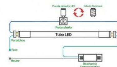
Diagrama de conexión conservando antigua instalación:
